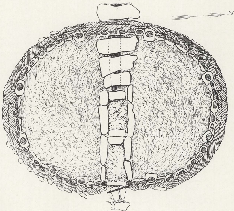
Fig. 17—18. Elias Jonassons näver- och torvtäckta bågstångskåta med bågstångskonstruktionen utbyggd (vidgad) med mellanstycke. På den breddade, ovala, golvplanen samma rumsindelning som i fig. 15—16 men med större luoito -utrymme. Den under fig. 14 nämnda lufttrumman till härden här markerad. Uppmätningsskisser av Arvid Hammarström 1943. Inre mått: bredd 420 cm, djup 320 cm, höjd till grytåsen 180 cm, till räppen (rököppningen) 260 cm.
