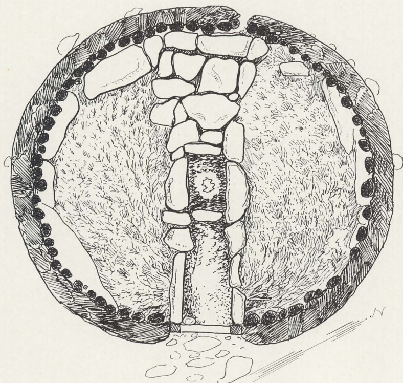
Fig. 15—16. Anders Torkelssons näver- och torvtäckta klykstångskåta med väggvirket mer eller mindre krumvuxet och inflätat i vartannat. I den nästan cirkelrunda golvplanen märks från dörren axeln ukes-arran-påssjo (förstugan-härden-köksavdelningen), delande luoito , det golvräckta utrymmet för kåtans folk. Uppmätningsskisser av Arvid Hammarström 1943. Inre mått: diam. ca 420 cm, höjd till klykkopplingen och räppen ca 230 cm.
