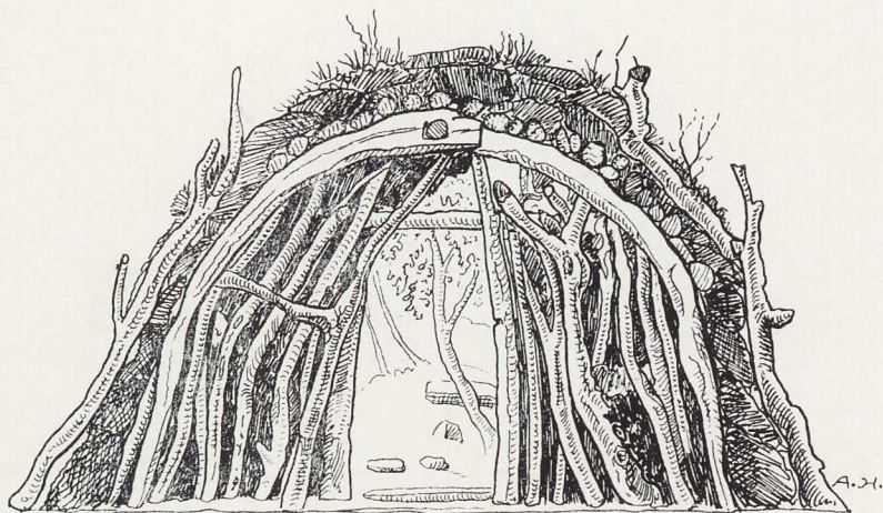
Fig. 19. Källarliknande förrådsåta tillhörande Jonas Jonasson (c), med bågstängskonstruktion under kavel- och torvtäckningen, tvärgenomskärning. Inre mått: bredd (mellan bågstängerna) ca 250 cm, längd ca 300 cm, höjd till åsen 165 cm. Uppmätningsskiss av Arvid Hammarström 1943.
