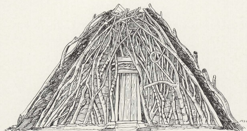
Fig. 15—16. Anders Torkelssons näver- och torvtäckta klykstångskåta med väggvirket mer eller mindre krumvuxet och inflätat i vartannat. I den nästan cirkelrunda golvplanen märks från dörren axeln ukes-arran-påssjo (förstugan-härden-köksavdelningen), delande luoito , det golvräckta utrymmet för kåtans folk. Uppmätningsskisser av Arvid Hammarström 1943. Inre mått: diam. ca 420 cm, höjd till klykkopplingen och räppen ca 230 cm.
