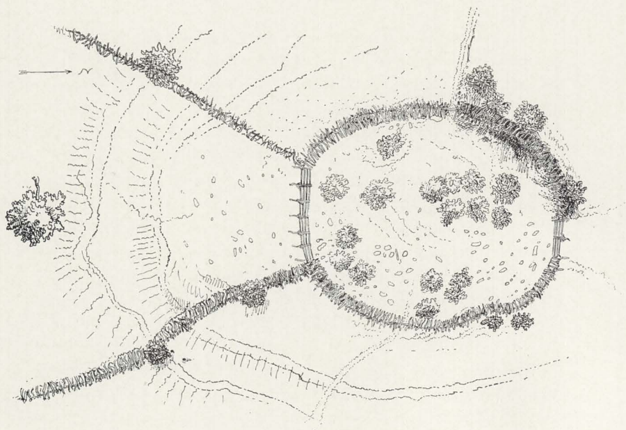
Fig. 22. Det äldre rengärdet vid Kroktjärnvallen, "klabbgärda" av den traditionella konstruktionen med lösa stockar lutade mot en horisontell, på klykkopplingar vilande slana. Fångstarmar (här tecknade den närmaste biten) leder mot inkörsgrinden; mitt emot en utsläppsgrind. Hagens längd 70 m, bredd 59. Skiss av Arvid Hammarström 1943.
