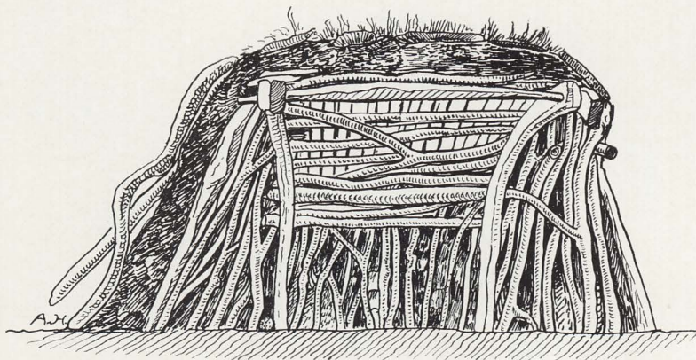
Fig. 20. Samma åta som fig. 19, längdgenomskärning. Uppmätningsskiss av Arvid Hammarström 1943.
