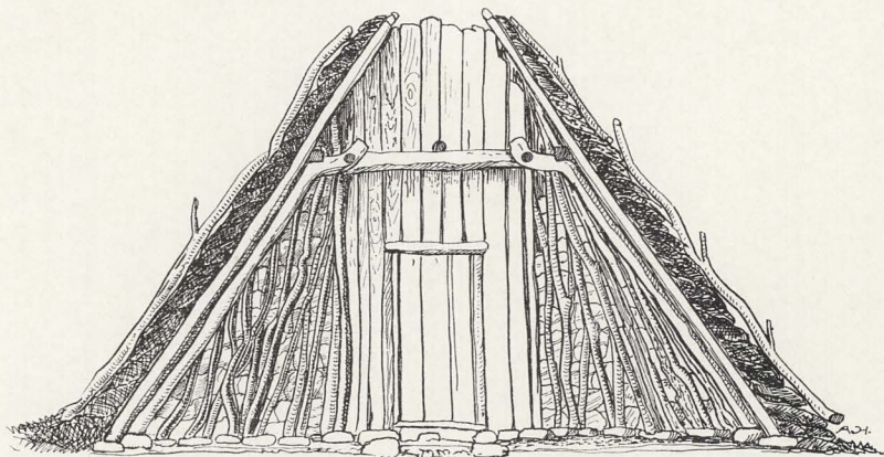
Fig. 17—18. Elias Jonassons näver- och torvtäckta bågstångskåta med bågstångskonstruktionen utbyggd (vidgad) med mellanstycke. På den breddade, ovala, golvplanen samma rumsindelning som i fig. 15—16 men med större luoito -utrymme. Den under fig. 14 nämnda lufttrumman till härden här markerad. Uppmätningsskisser av Arvid Hammarström 1943. Inre mått: bredd 420 cm, djup 320 cm, höjd till grytåsen 180 cm, till räppen (rököppningen) 260 cm.
