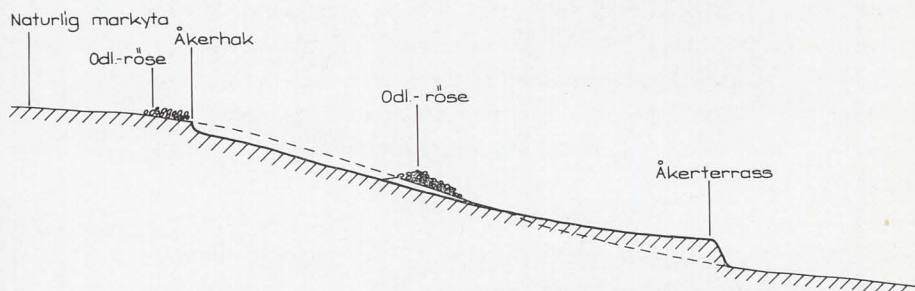
Bild 1. Principskiss i profil över en fossil åkers uppkomst och utseende. Jord föres genom odlingen från sluttningens högre del mot den nedre, där åkerterrassen uppkommer i kanten. I övre kanten bildas däremot ett åkerhak. Odlingsrösen kan ligga som impediment i åkern eller vara uppkastade omedelbart invid dennas kanter.
